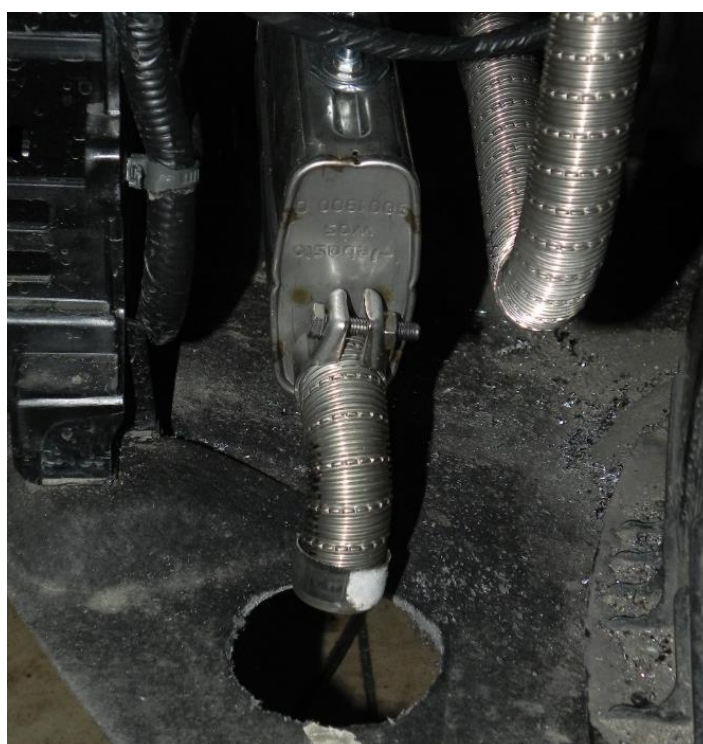
tłumik wydechu
