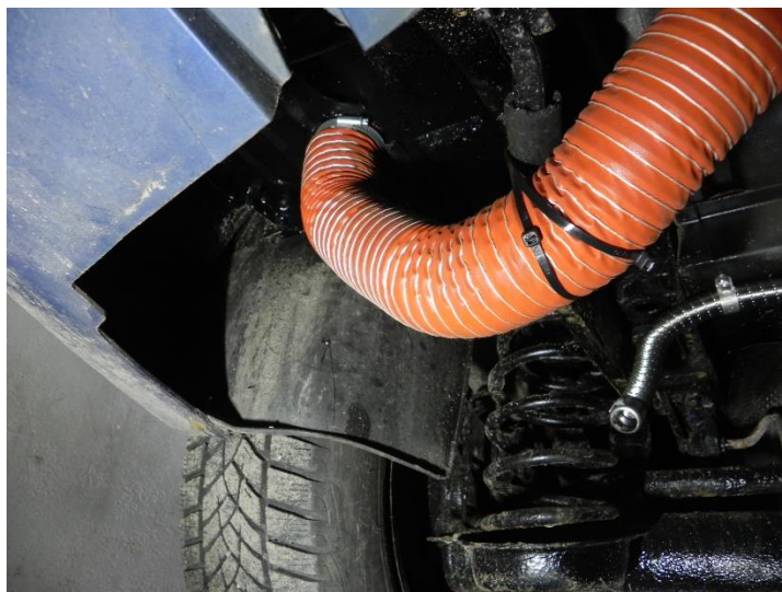
rura dystrybucji powietrza i rura wydechu
