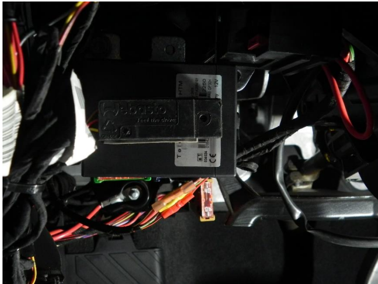
odbiornik Telestart / czujnik temperatury
