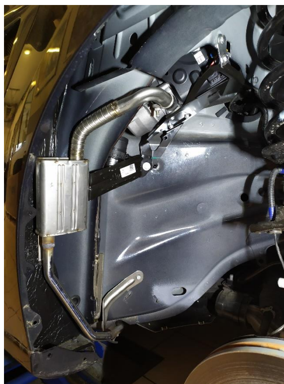
agregat / wydech
