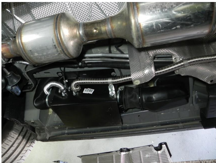
łapa agregatu, wylot powietrza ogrzanego
